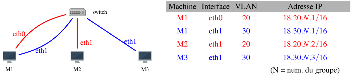
FIGURE 1 – Une première solution de routage avec une interface par VLAN sur M1
